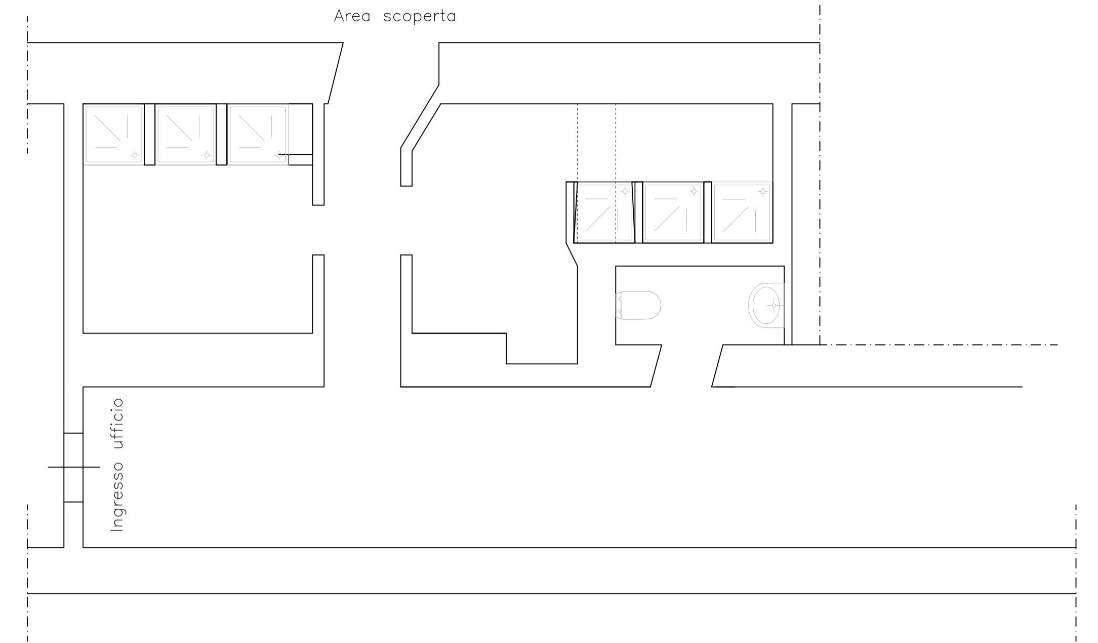
NUOVO LAYOUT DOCCE/WC Scala 1:50
