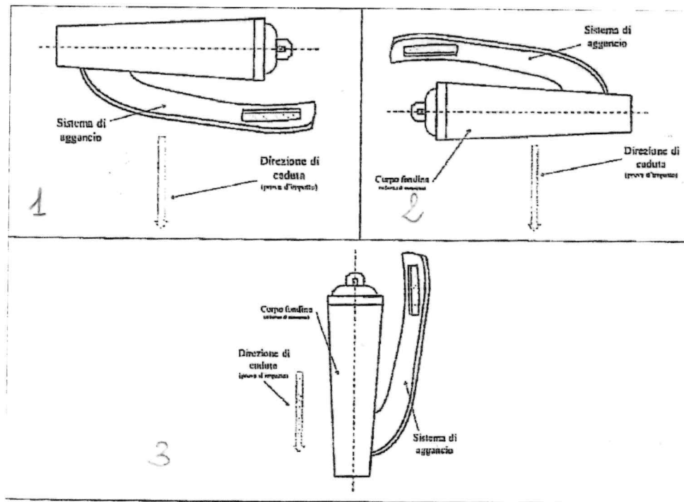
Figura 4: schemi di caduta
