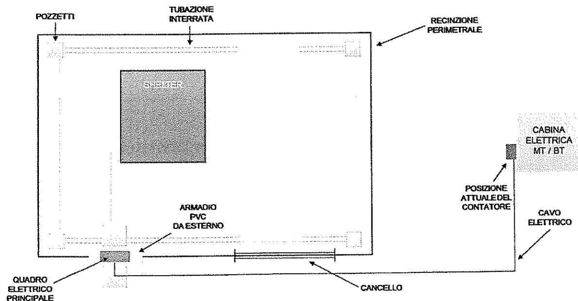
Figura 3 – Schema attuale del sito
