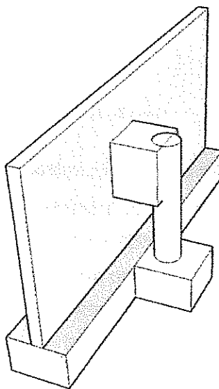
Figura 10 – Montaggio del palo e taglio recinzione
