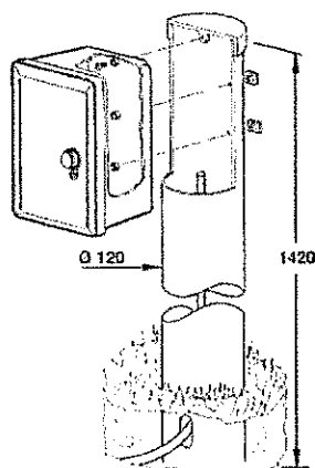
Installazione armadio
