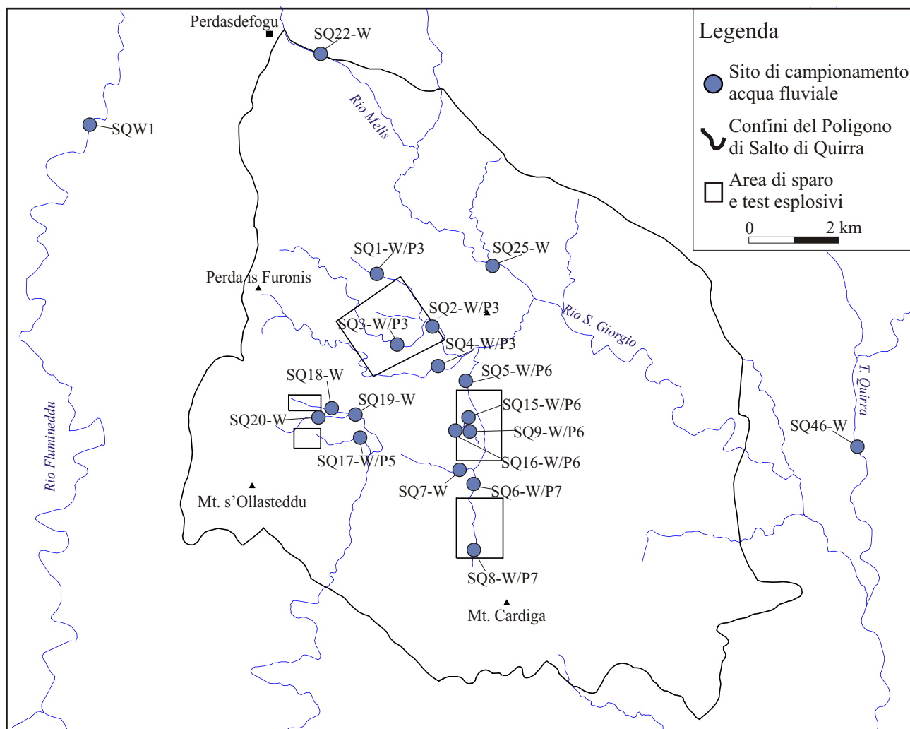
Fig. 10.1. Ubicazione dei campioni di acqua fluviale prelevati nell'area del Poligono di Perdasdefogu.
