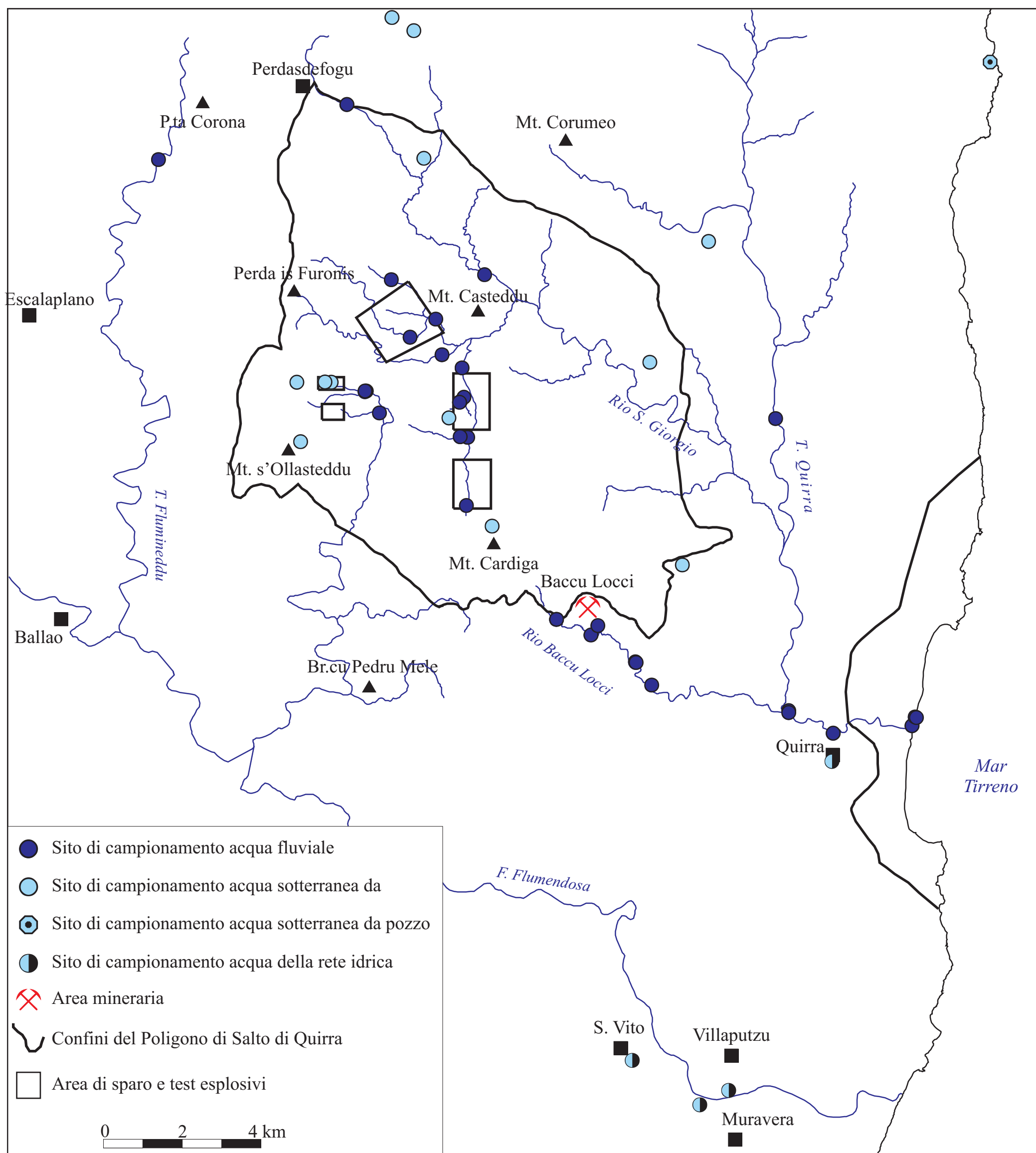
Fig. 3.4. Ubicazione dei siti di prelievo di campioni di acque fluviali e sotterranee nell'area del Salto di Quirra.
