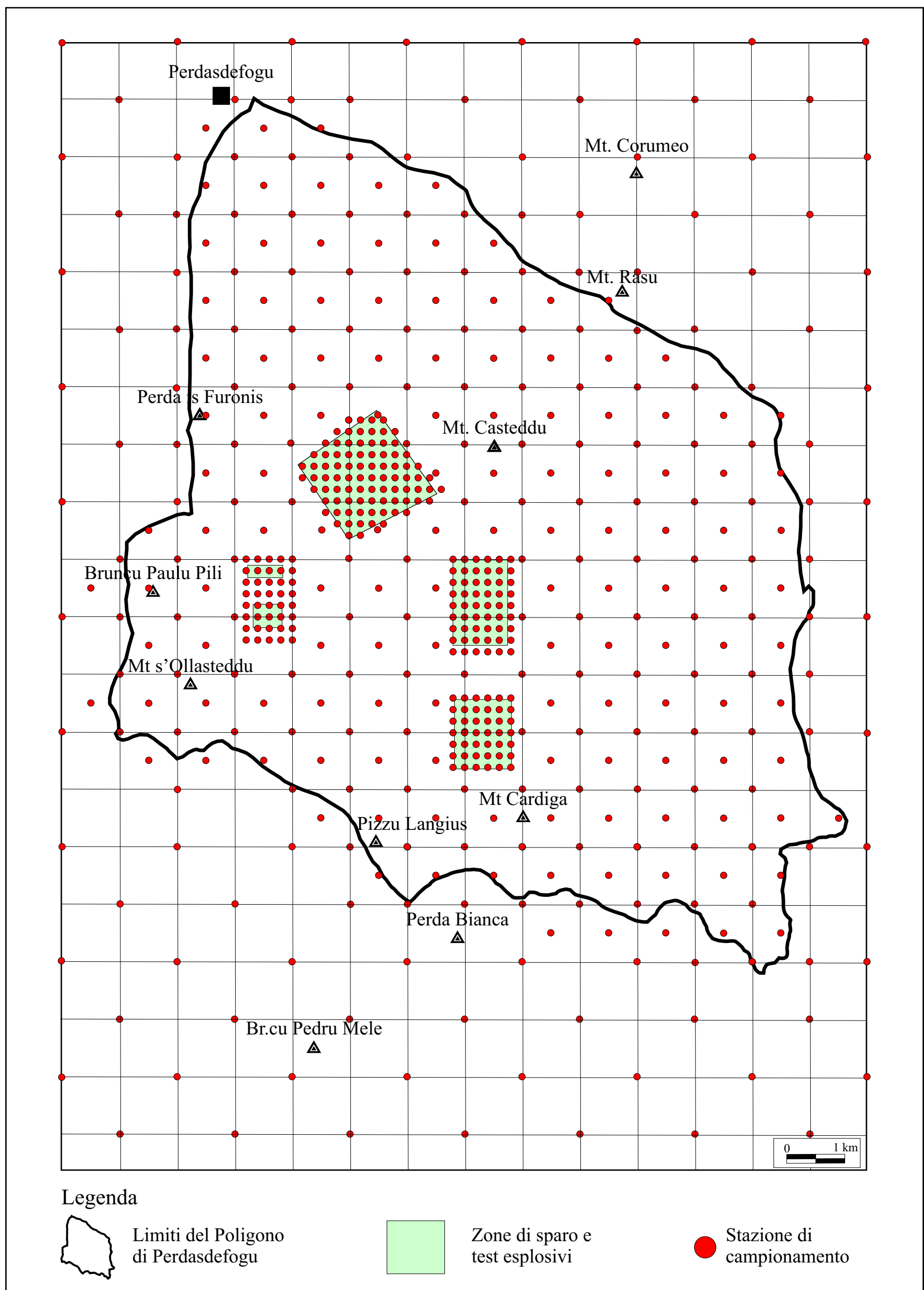
Fig. 3.7. Strategia e piano di campionamento di suoli nell'area del Poligono di Perdasdefogu.
