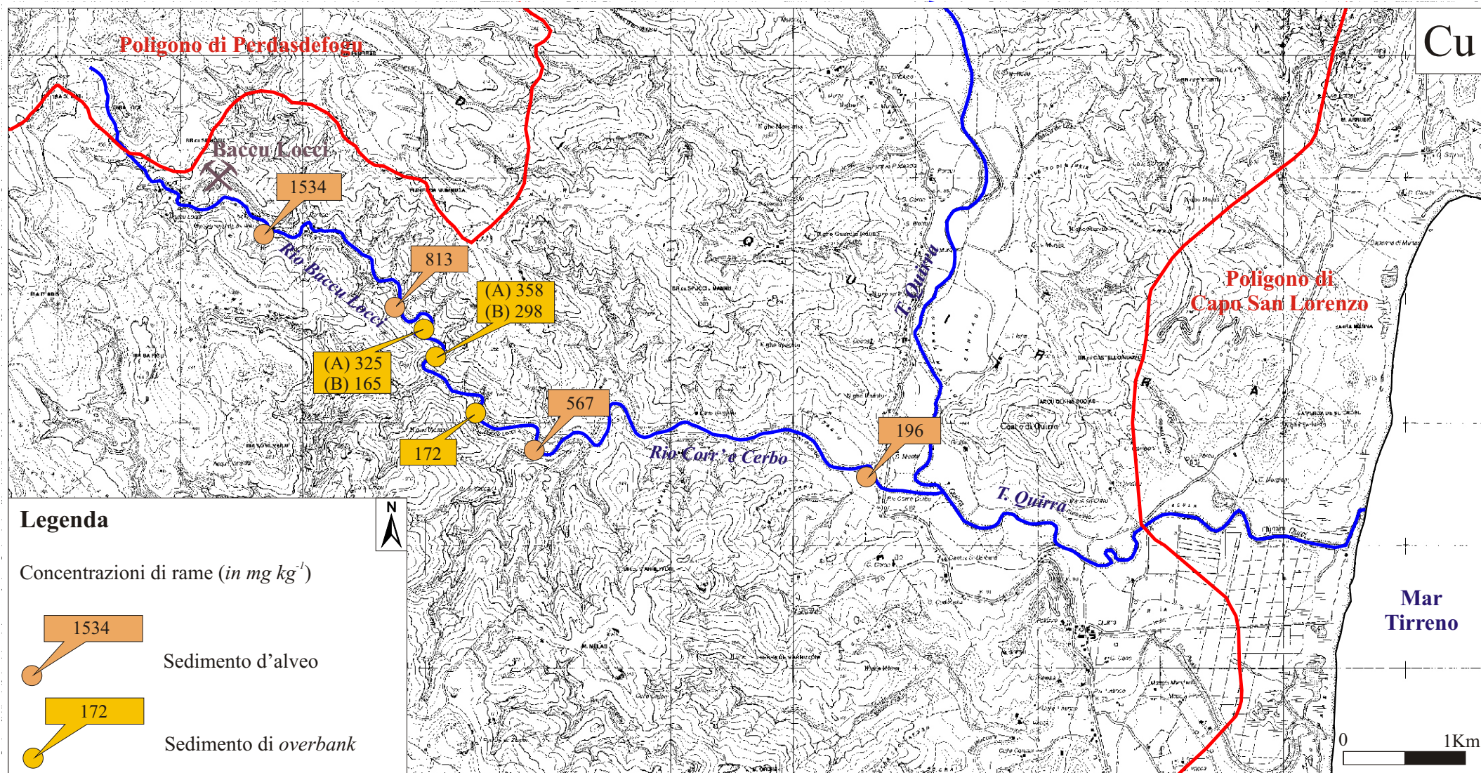
Fig. 11.9. Concentrazioni di rame nei campioni di sedimento fluviale prelevati nel sistema idrografico Rio Baccu Locci - Rio Corr'e Cerbo.
