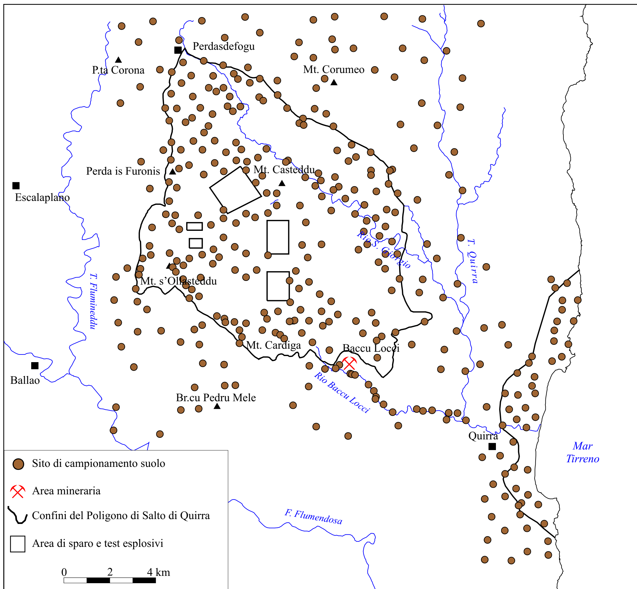
Fig. 3.2. Ubicazione dei siti di prelievo di campioni di suolo nell'area del Salto di Quirra.
