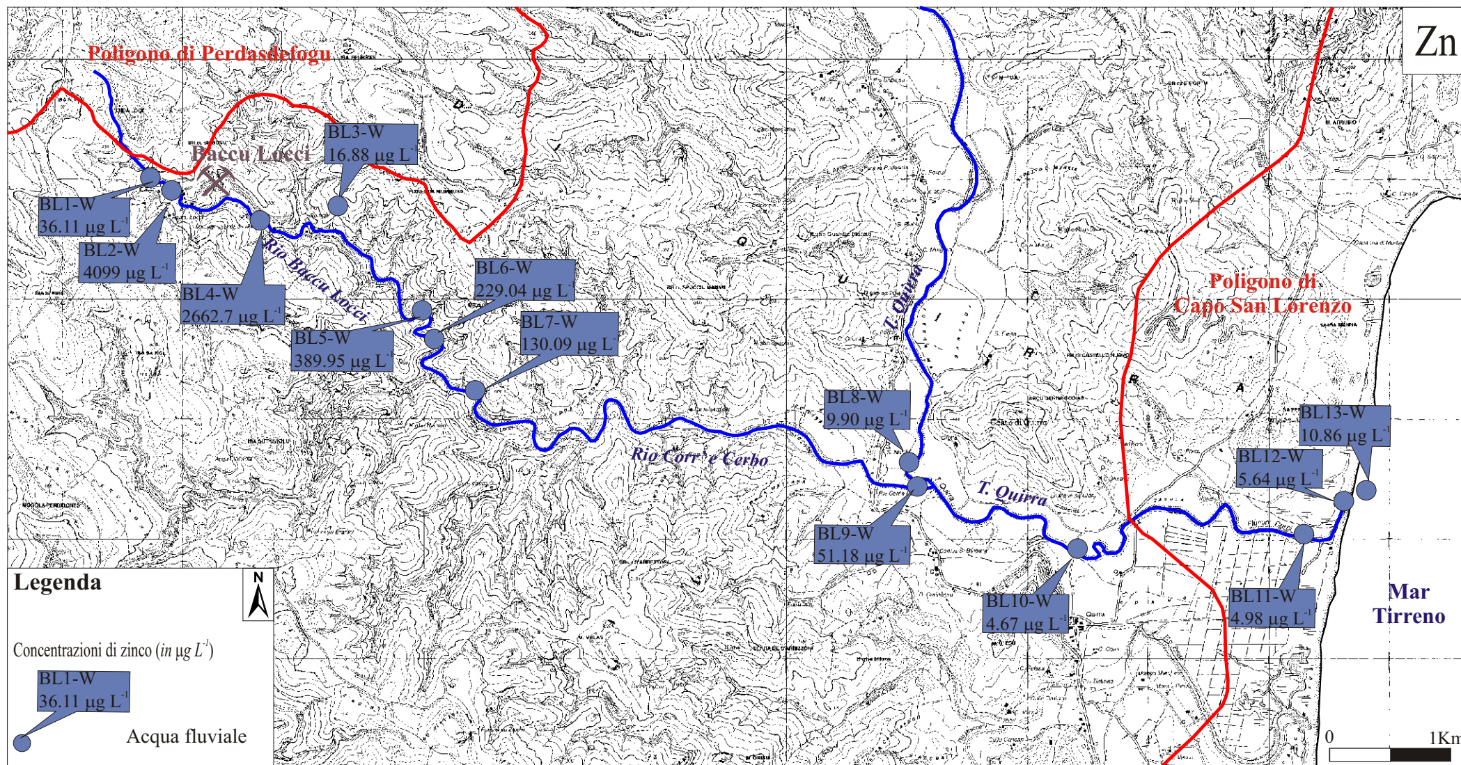
Fig. 10.7. Concentrazioni di zinco nei campioni di acqua fluviale prelevati nel sistema idrografico Rio Baccu Locci - Rio Corr'e Cerbo - T. Quirra.
