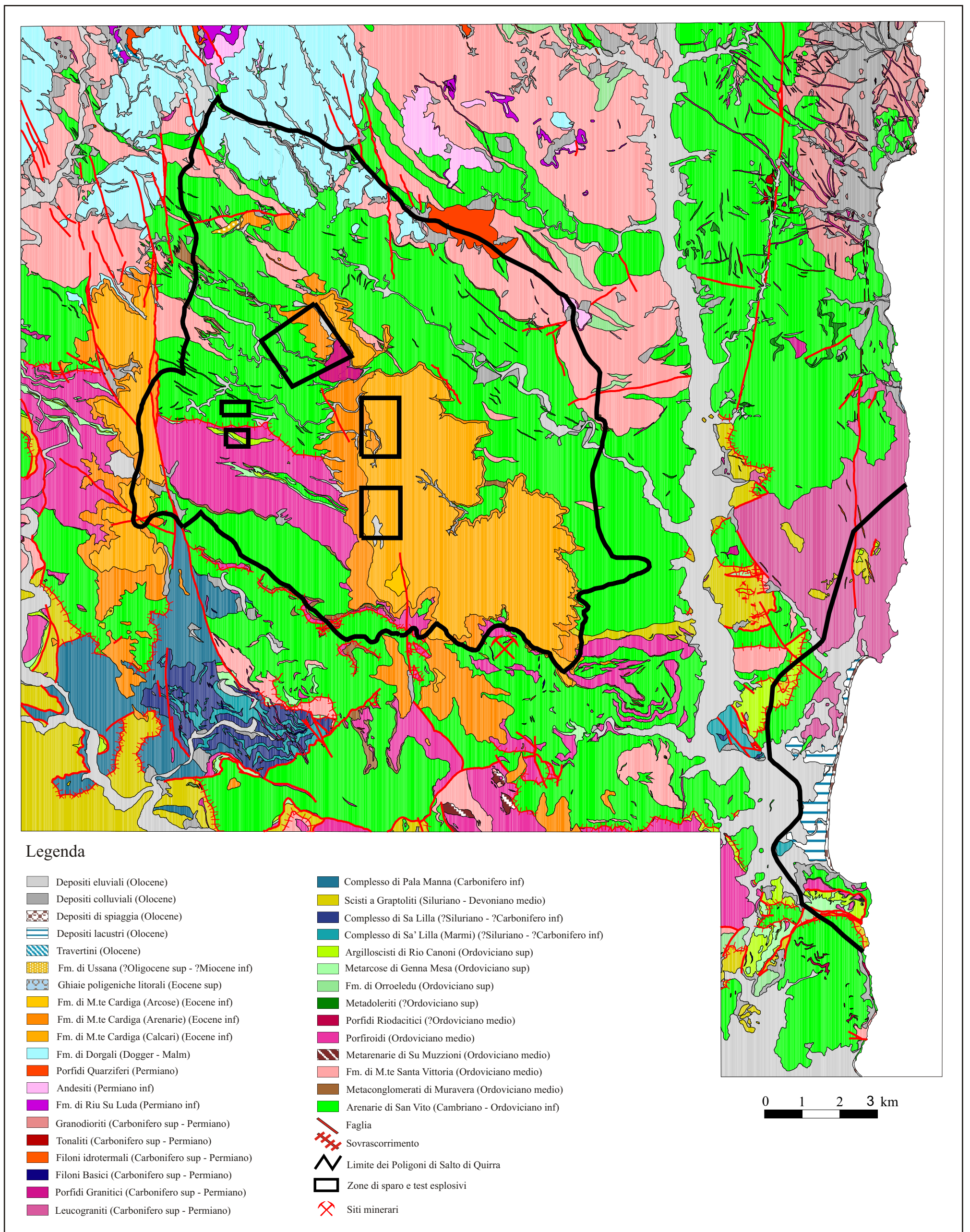
Fig. 2.4. Carta geologica dell'area del Salto di Quirra.
