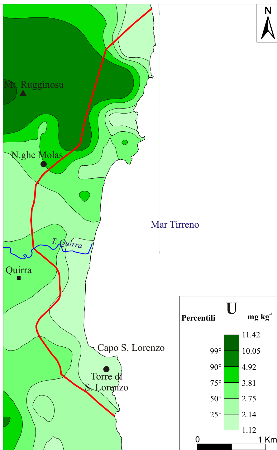
Fig. 9.29. Carta geochimica della distribuzione dell'uranio nei suoli dell'area del Poligono di Capo San Lorenzo.
